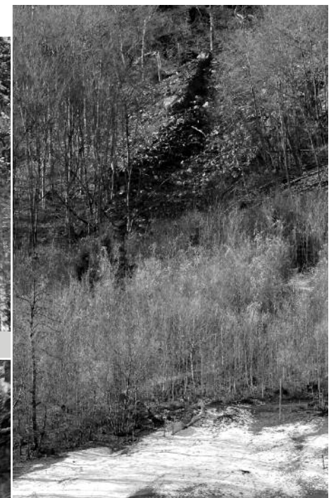
Der Schuttkegel über der Mugi, unten die Zäune des Skilifts. (Foto: Christian Bosshard)
